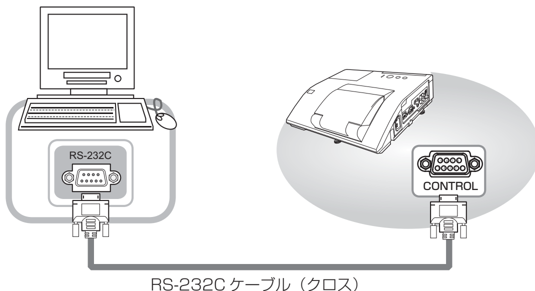
コンピュータの RS-232C 端子
